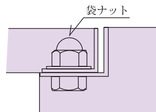
ボルト部詳細図
