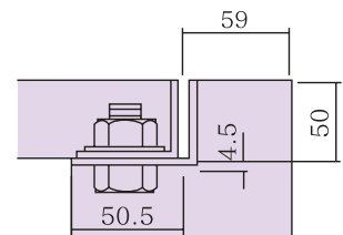
ボルト部詳細図
