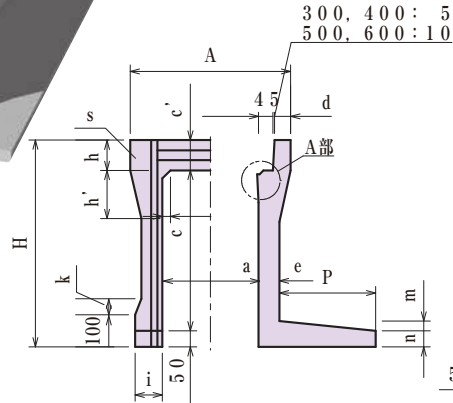
正面図
