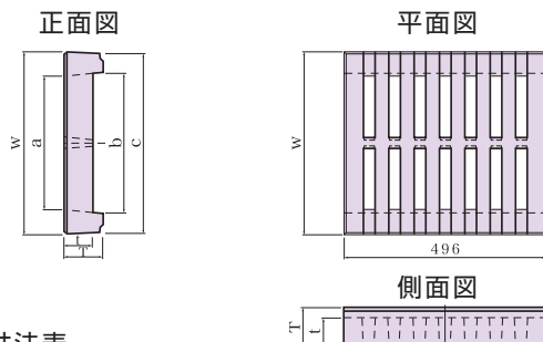
寸法表
