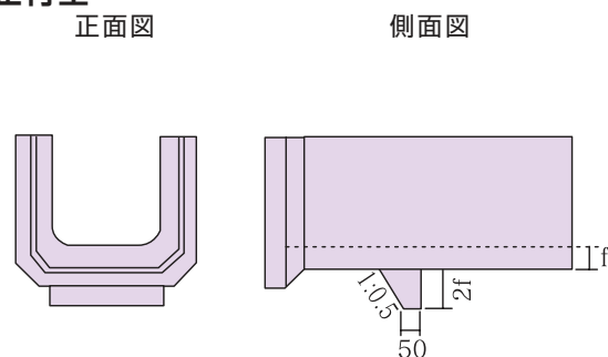
滑止付型
