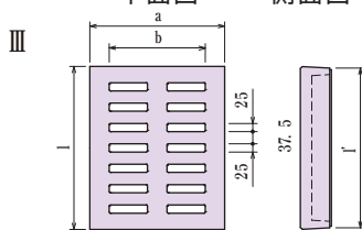
正面図
