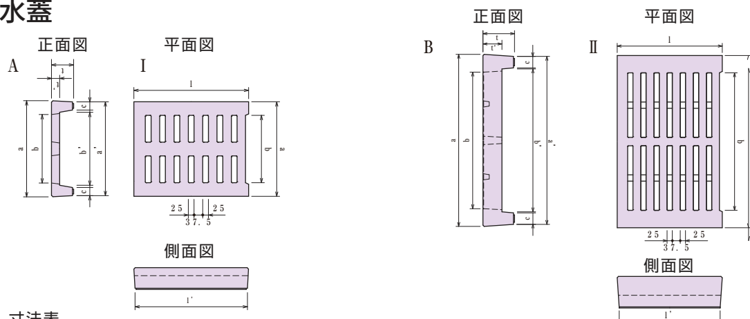
寸法表
