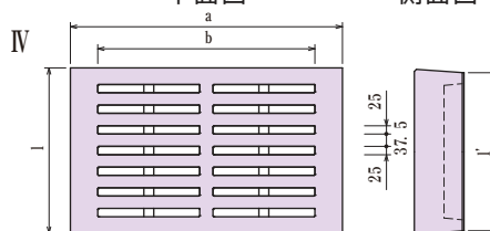
正面図
