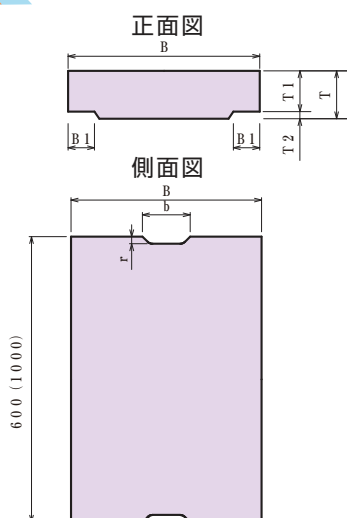
寸法表
