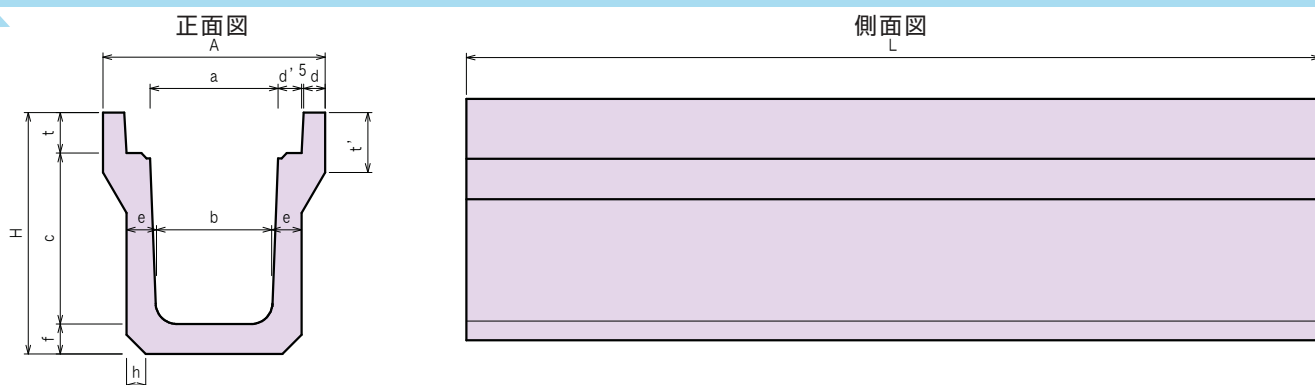
寸法表
