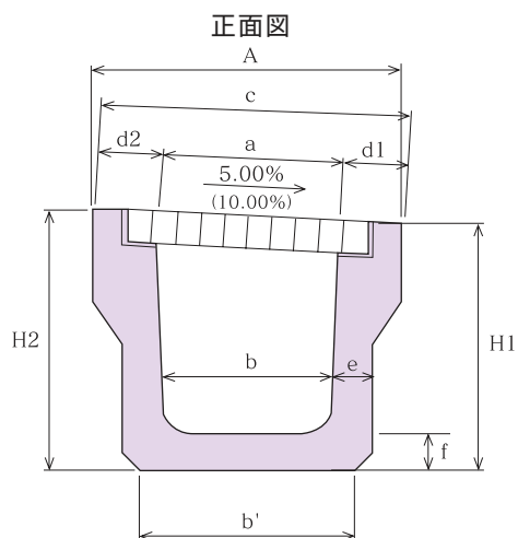
寸法表
