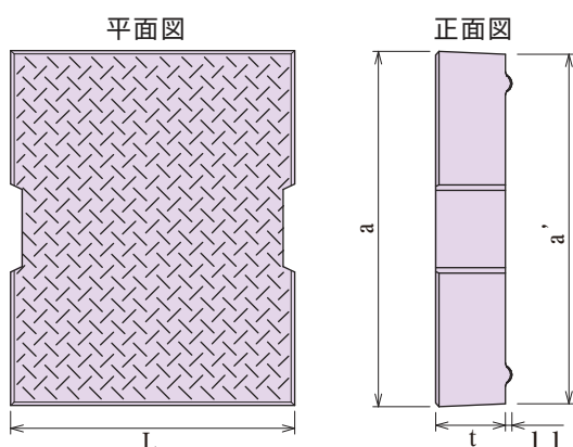
側溝蓋
