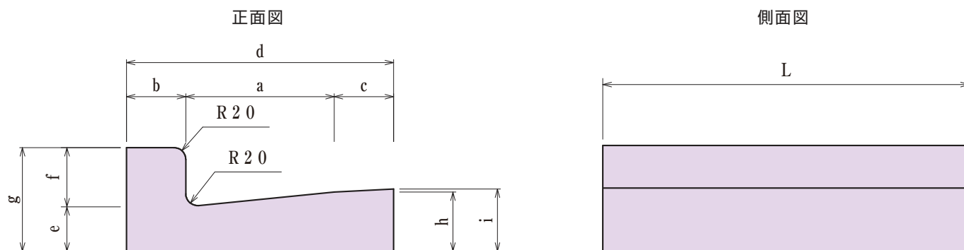
寸法表
