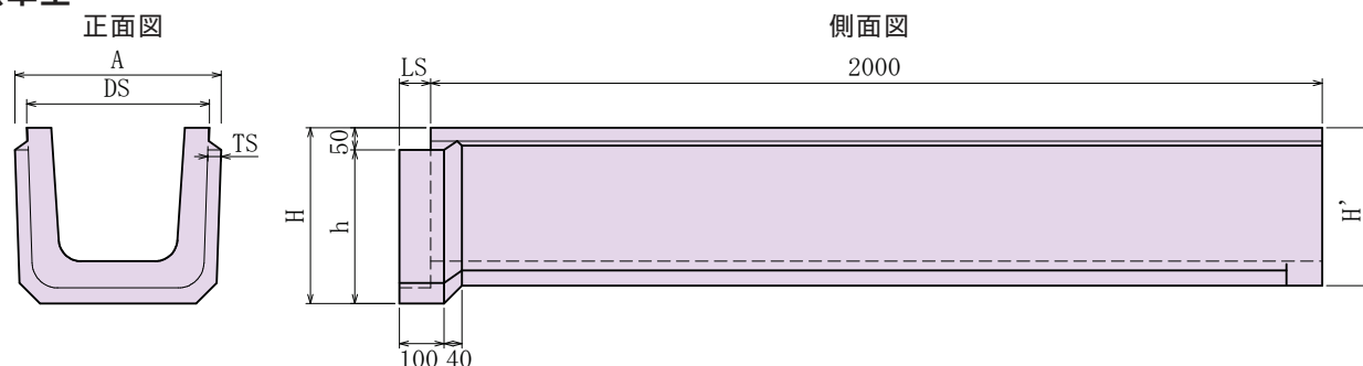
寸法表
