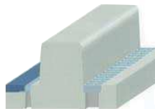
【3】縁石付き両面取水型 歩道側は15mm幅のスリット、車道側は60mmのグレーチング構造です。 一つの側溝で歩道を車道の両側から取水できます。
