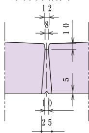
梁部詳細図
