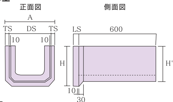
標準型
