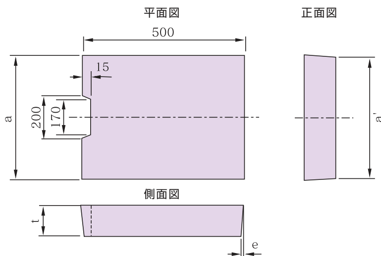
寸法表
