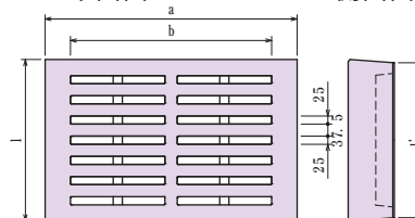
平面図
