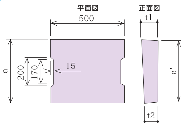
寸法表
