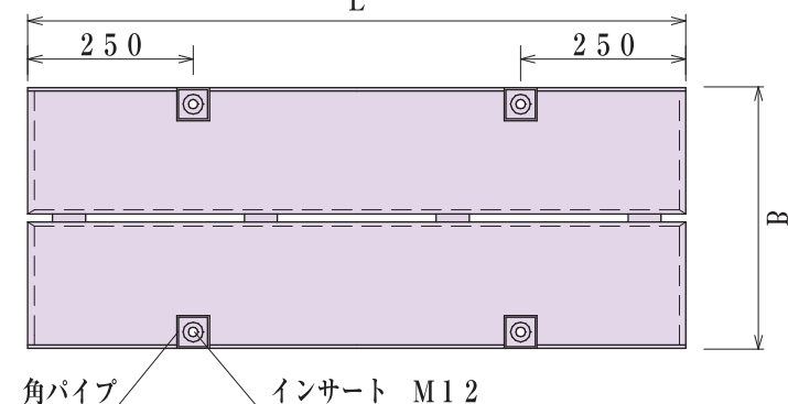
KS 側溝型側面図
