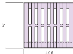
側面図
