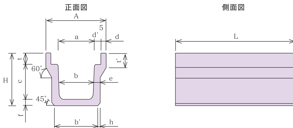
寸法表（車道用）
