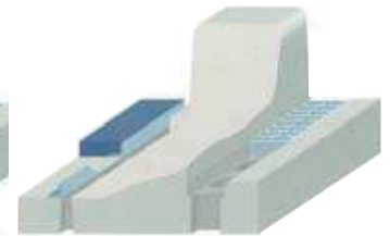
【3】縁石付き両面取水型 歩道側は15mm幅のスリット、車道側は60mmのグレーチング構造です。 一つの側溝で歩道を車道の両側から取水できます。
