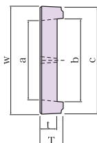
正面図
