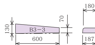
B片R～B片R〔乗入〕（3段下り-3）・左右 H=70 26kg
