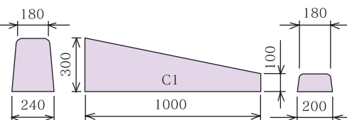
C両R～C両R(1段下り)
