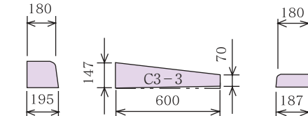
C片R～C片R〔乗入〕（3段下り-3）・左右 H=70
