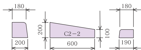
C片R～C片R〔乗入〕（2段下り-2）・左右
