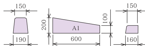
A両R～A片R〔乗入〕(1段下り)・左右
