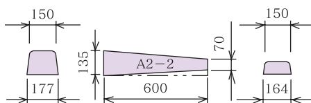
A両R～A両R(2段下り-2)
