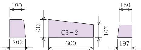
C片R～C片R〔乗入〕（3段下り-2）・左右
