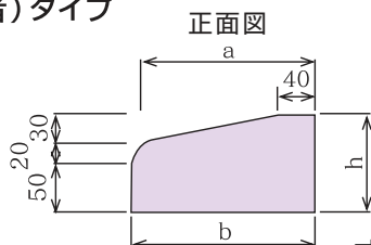
片面(身障者)タイプ
