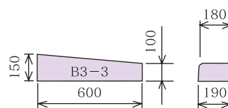
B片R～B片R〔乗入〕（3段下り-3）・左右 33kg
