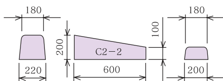
C両R～C両R(2段下り-2)・左右
