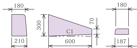
C片R～C片R〔乗入〕（1段下り）・左右 H=70
