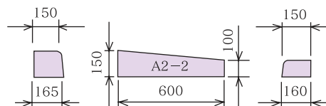
A片R～A片R〔乗入〕(2段下り-2)・左右
