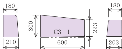
C片R～C片R〔乗入〕（3段下り-1）・左右 H=70
