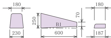
B両R～B片R(乗入)(1段下り)・左右 H=70
