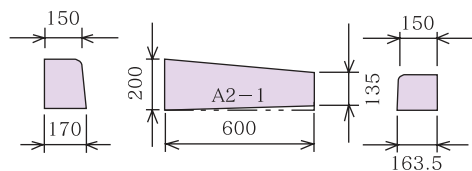
A片R～A片R〔乗入〕(2段下り-1)・左右 H=70
