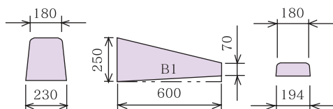
B両R～B両R(1段下り) H=70
