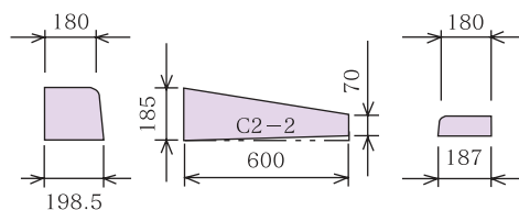
C片R～C片R〔乗入〕（2段下り-2）・左右 H=70
