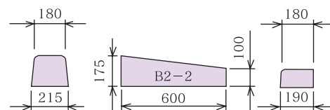
B両R～B片R(乗入)(2段下り-2)・左右
