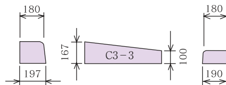
C片R～C片R〔乗入〕（3段下り-3）・左右
