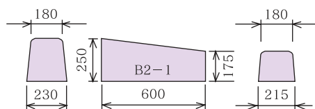
B両R～B両R(2段下り-1)
