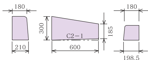
C片R～C片R〔乗入〕（2段下り-1）・左右 H=70
