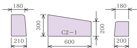
C片R～C片R〔乗入〕（2段下り-1）・左右
