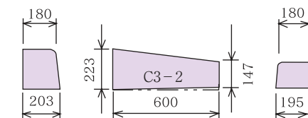
C片R～C片R〔乗入〕（3段下り-2）・左右 H=70
