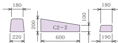
C両R～C片R〔乗入〕(2段下り-2)・左右
