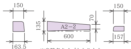
A片R～A片R〔乗入〕(2段下り-2)・左右 H=70
