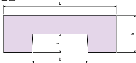
側面図
