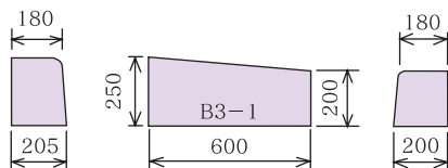
B片R～B片R〔乗入〕（3段下り-1）・左右 62kg
