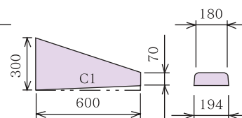
C両R～C両R(1段下り) H=70
