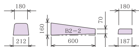
B両R～B片R(乗入)(2段下り-2)・左右 H=70
