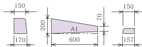
A片R～A片R〔乗入〕(1段下り)・左右 H=70
