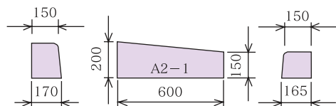
A片R～A片R〔乗入〕(2段下り-1)・左右
