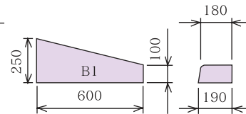
B両R～B片R(乗入)(1段下り)・左右
