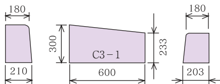
C片R～C片R〔乗入〕（3段下り-1）・左右
