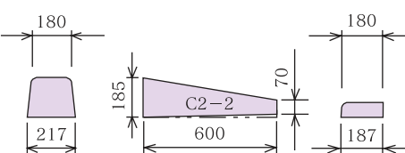
C両R～C片R〔乗入〕(2段下り-2)・左右 H=70
