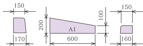
A片R～A片R〔乗入〕(1段下り)・左右
