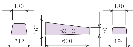
B両R～B両R(2段下り-2) H=70
