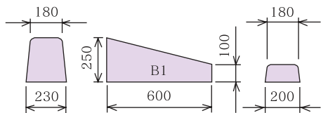
B両R～B両R(1段下り)
