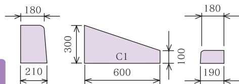
C片R～C片R〔乗入〕（1段下り）・左右
