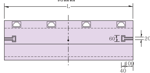
側面図
